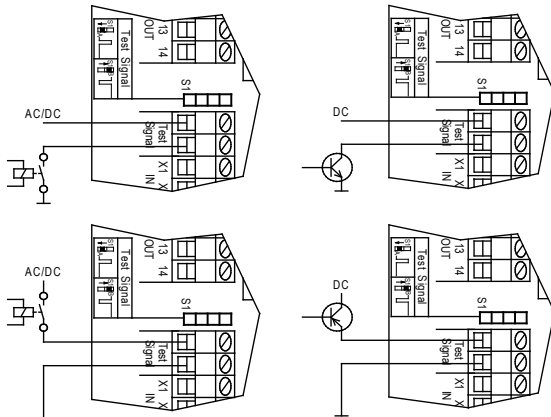
Anschlussklemmen Testsignal
