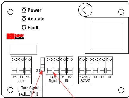
DIP-Schiebeschalter S1
